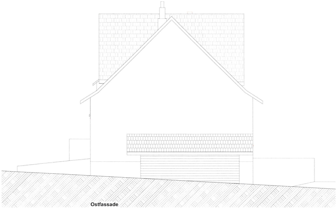
Ostfassade
