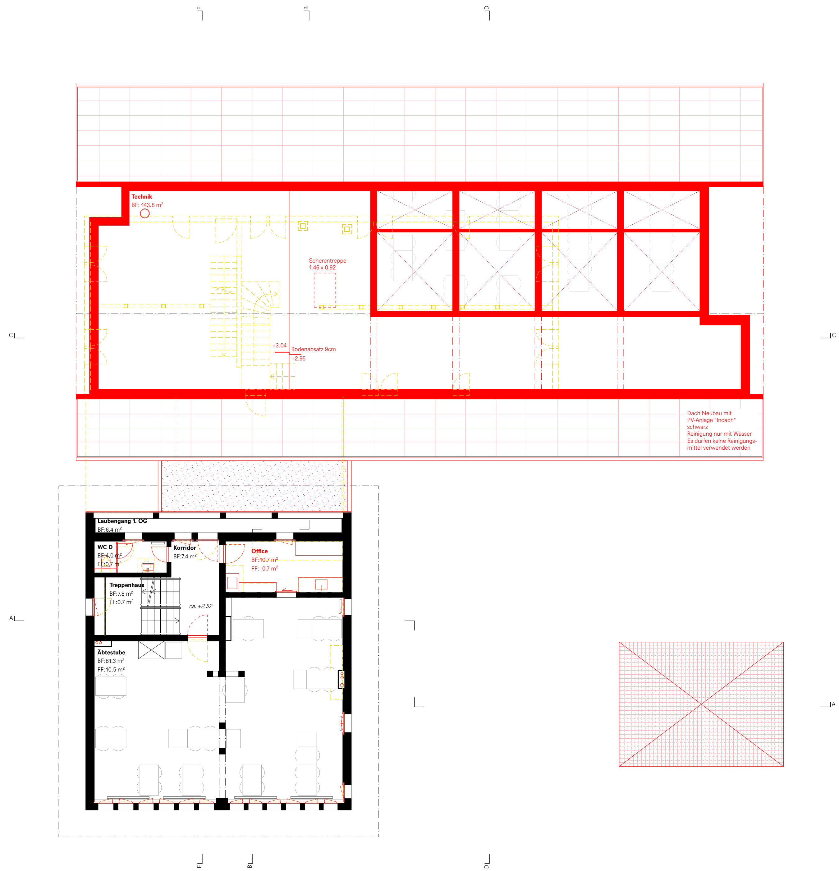
Grundriss 1. Obergeschoss
