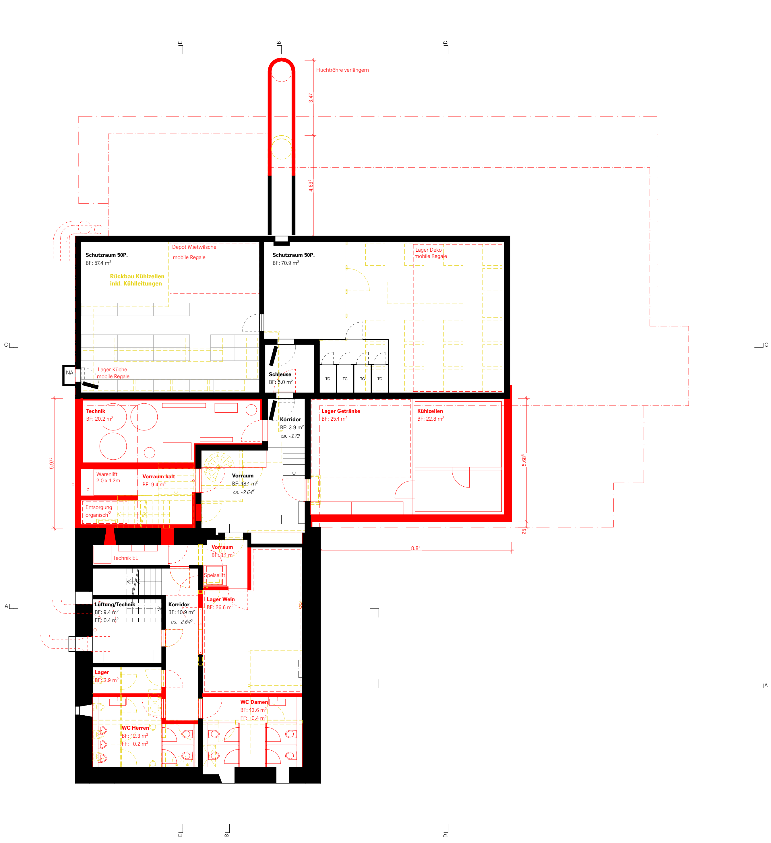
Grundriss Untergeschoss
