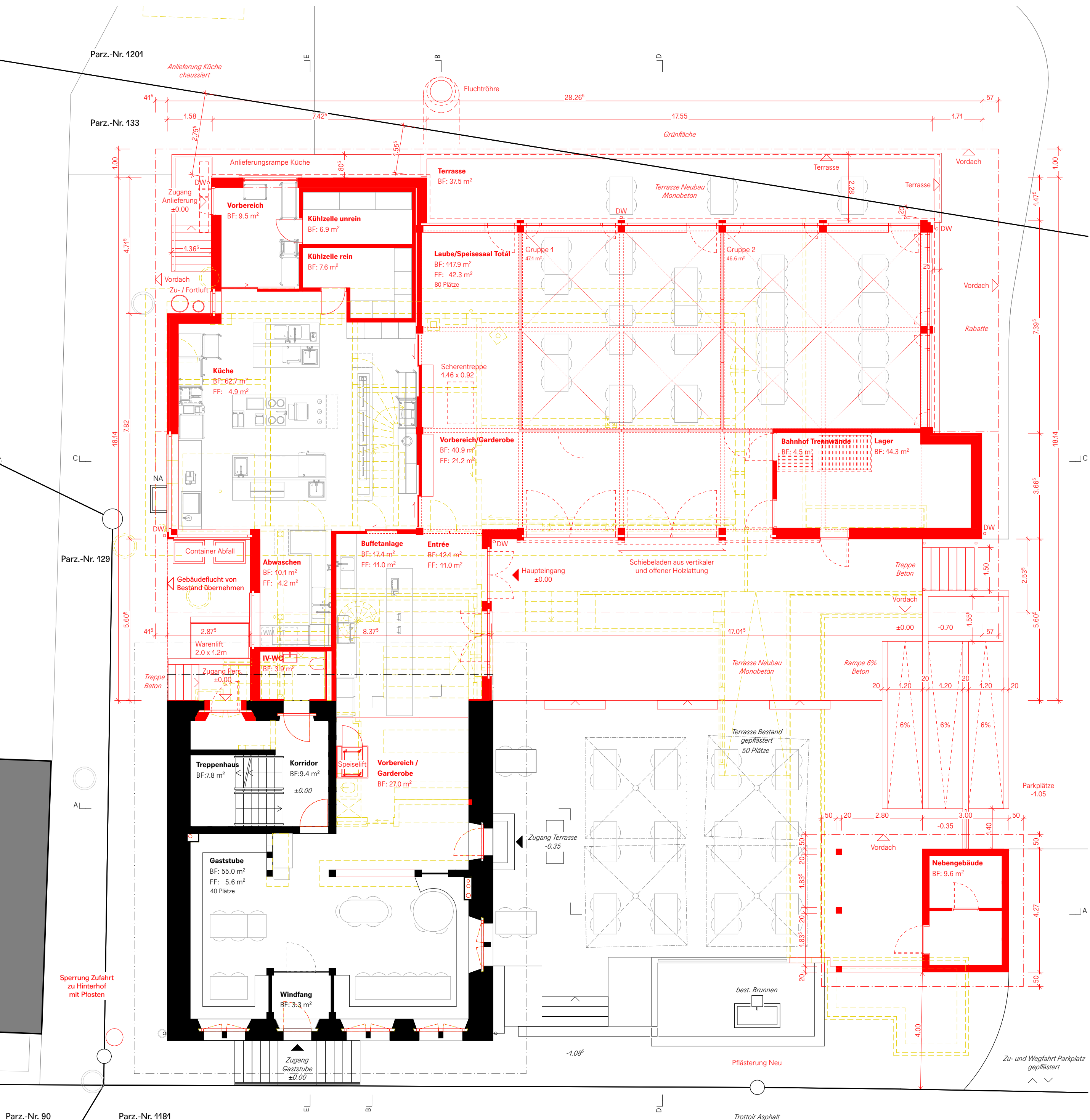
Grundriss Erdgeschoss mit Umgebung
