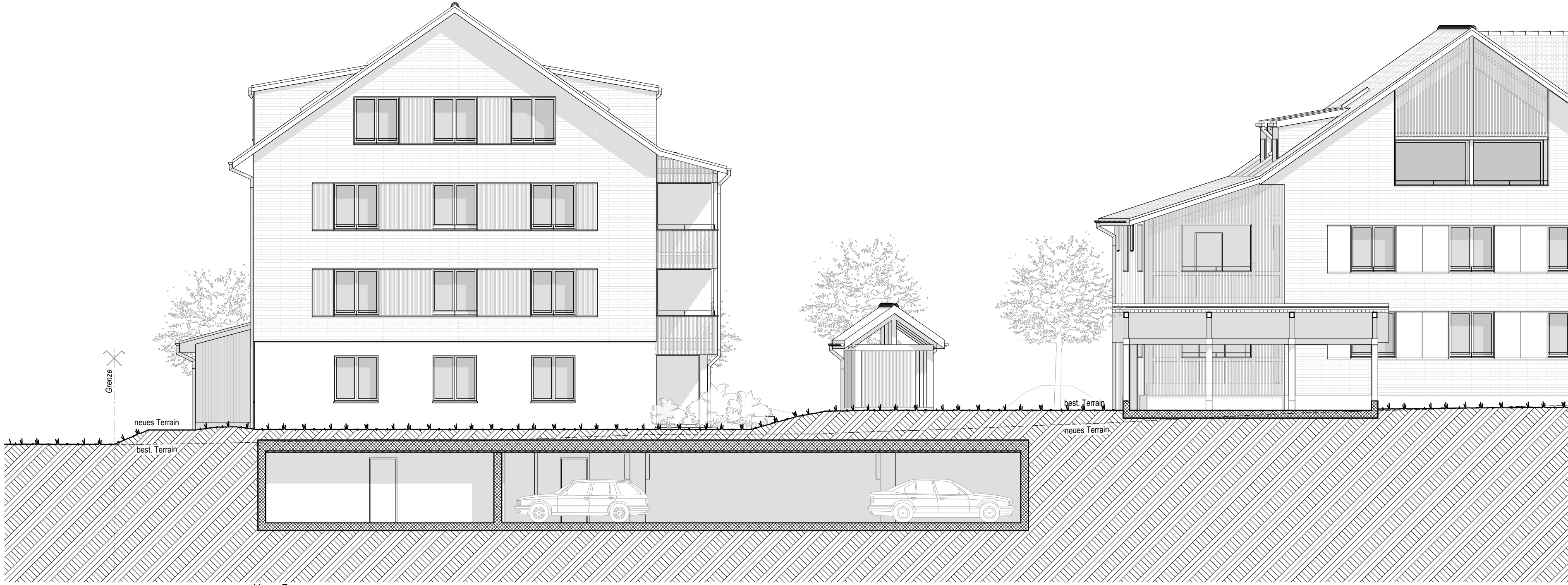
Haus B Süd-Westfassade 1:100
