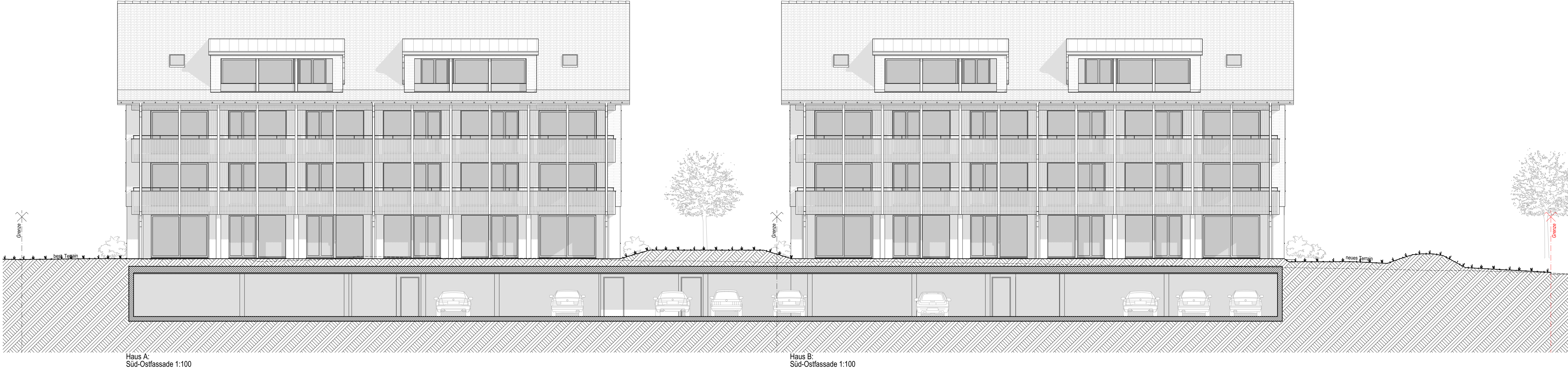
Haus A Süd-Ostfassade 1:100
