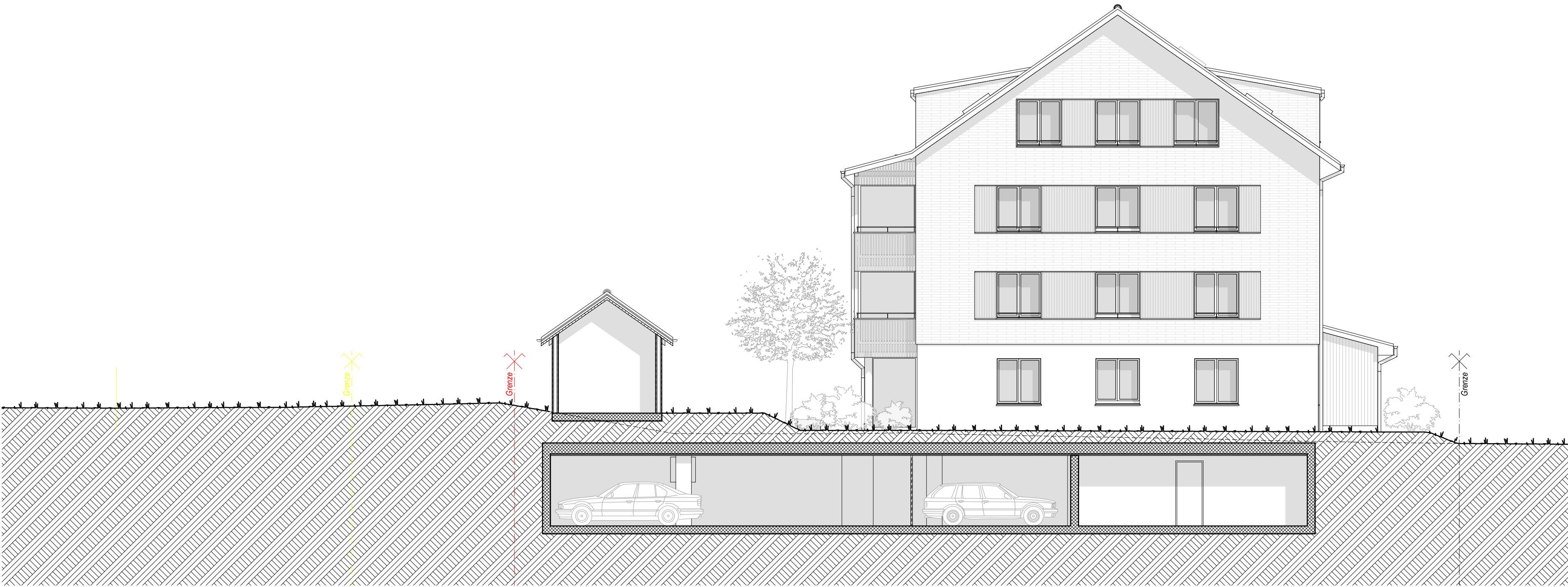
Haus A Nord-Ostfassade 1:100
