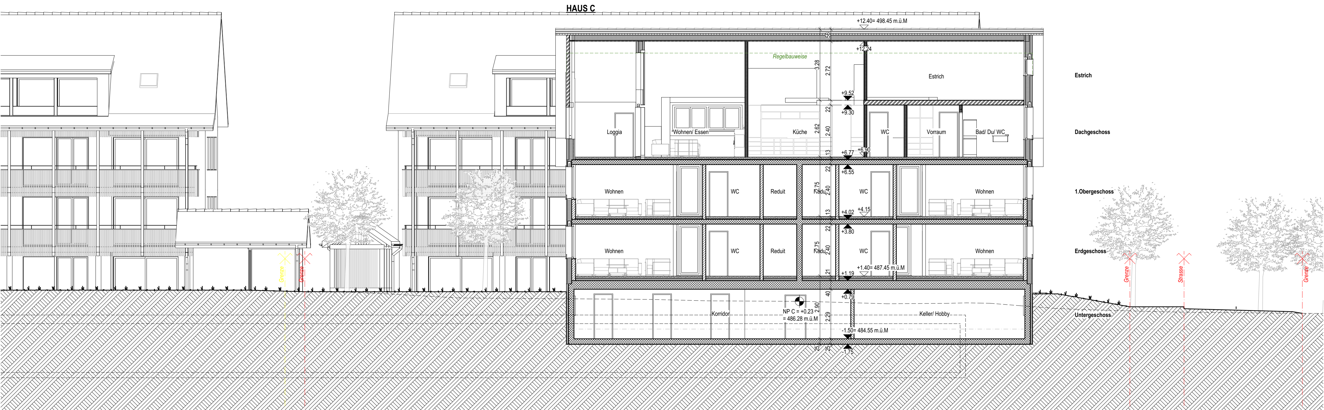
Haus C: Längsschnitt 1:100
