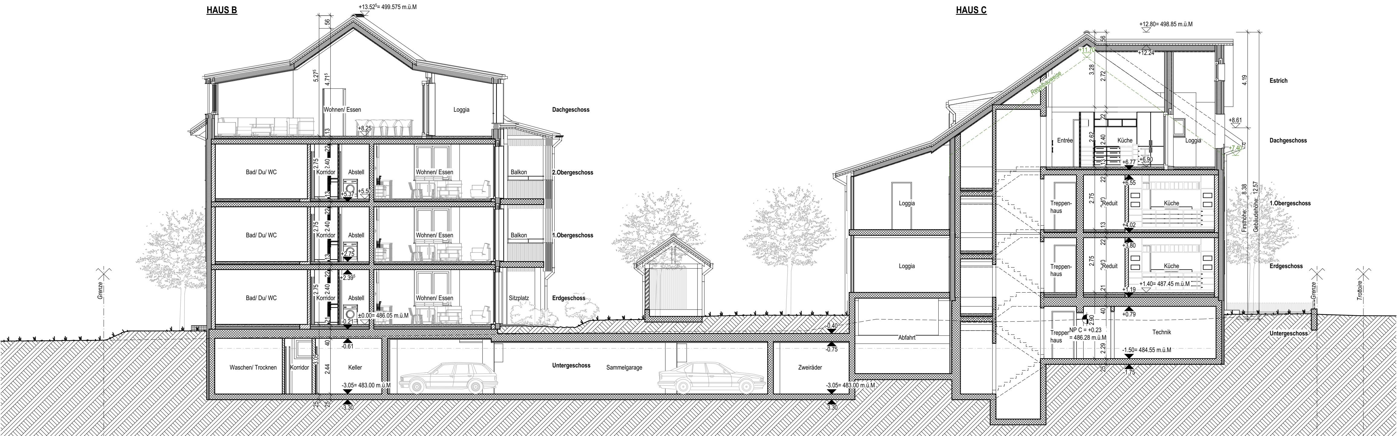
Haus C: Querschnitt 1:100
