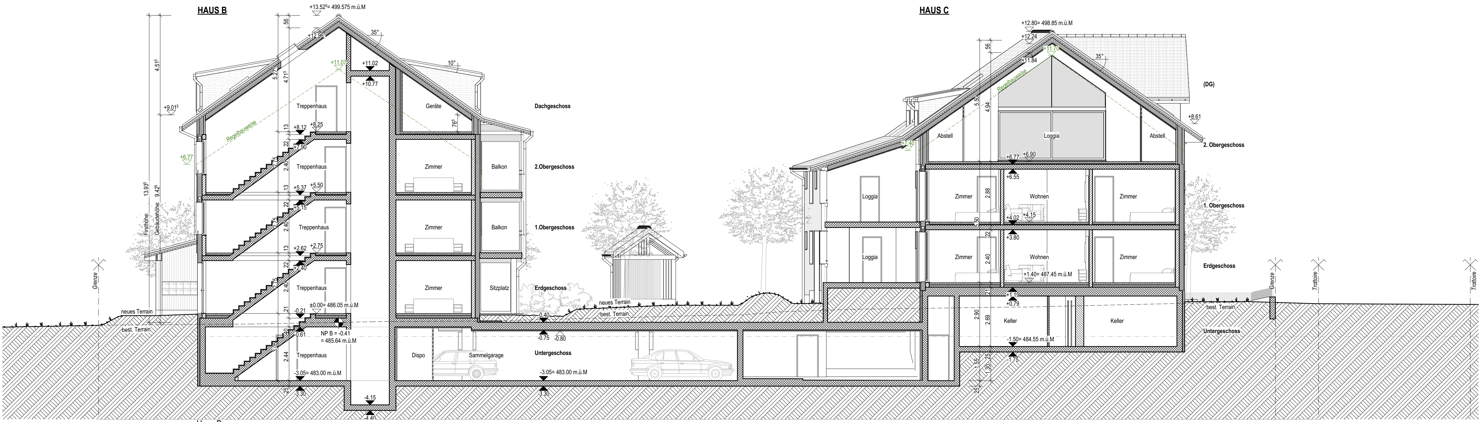
Haus B: Querschnitt 1:100
