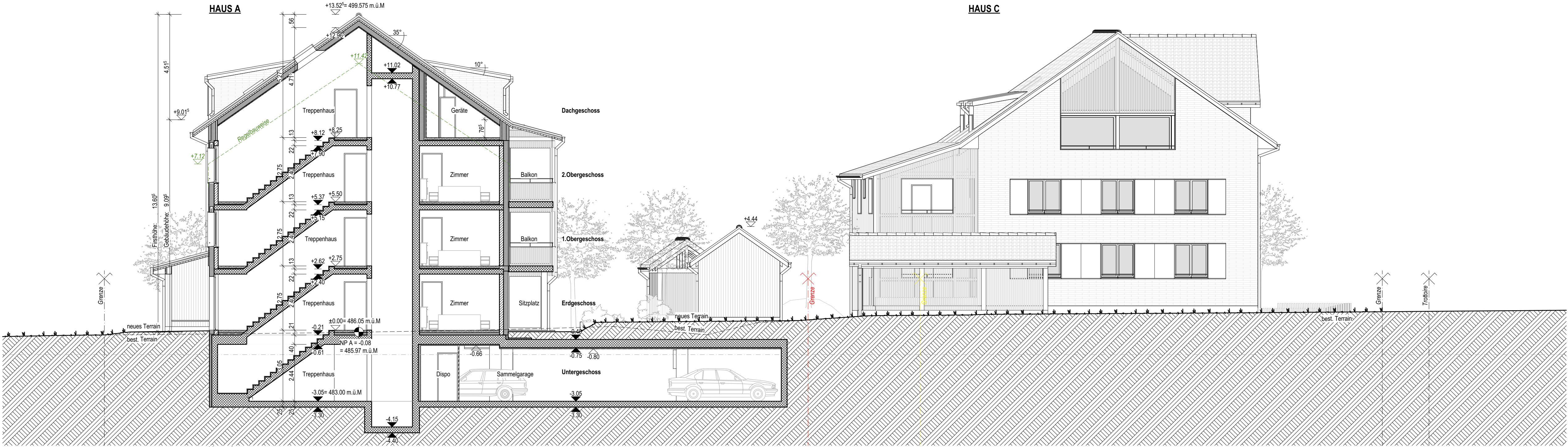
Haus A: Querschnitt 1:100
