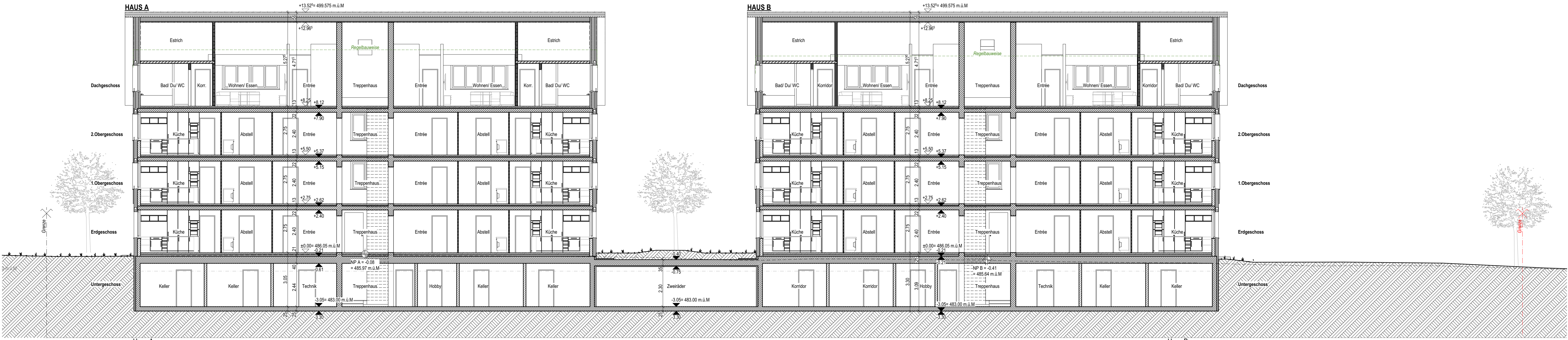
Haus A: Längsschnitt 1:100
